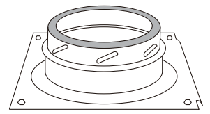
H :1x Verankerungsplatte H :1x Anchor plate H :1x Support de base H :1x Bevestigingsplaat
