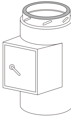
C :1x T-Anschluss 90 C :1x Inspection length C :1x Trappe de ramonage C :1x Inspectieluik
